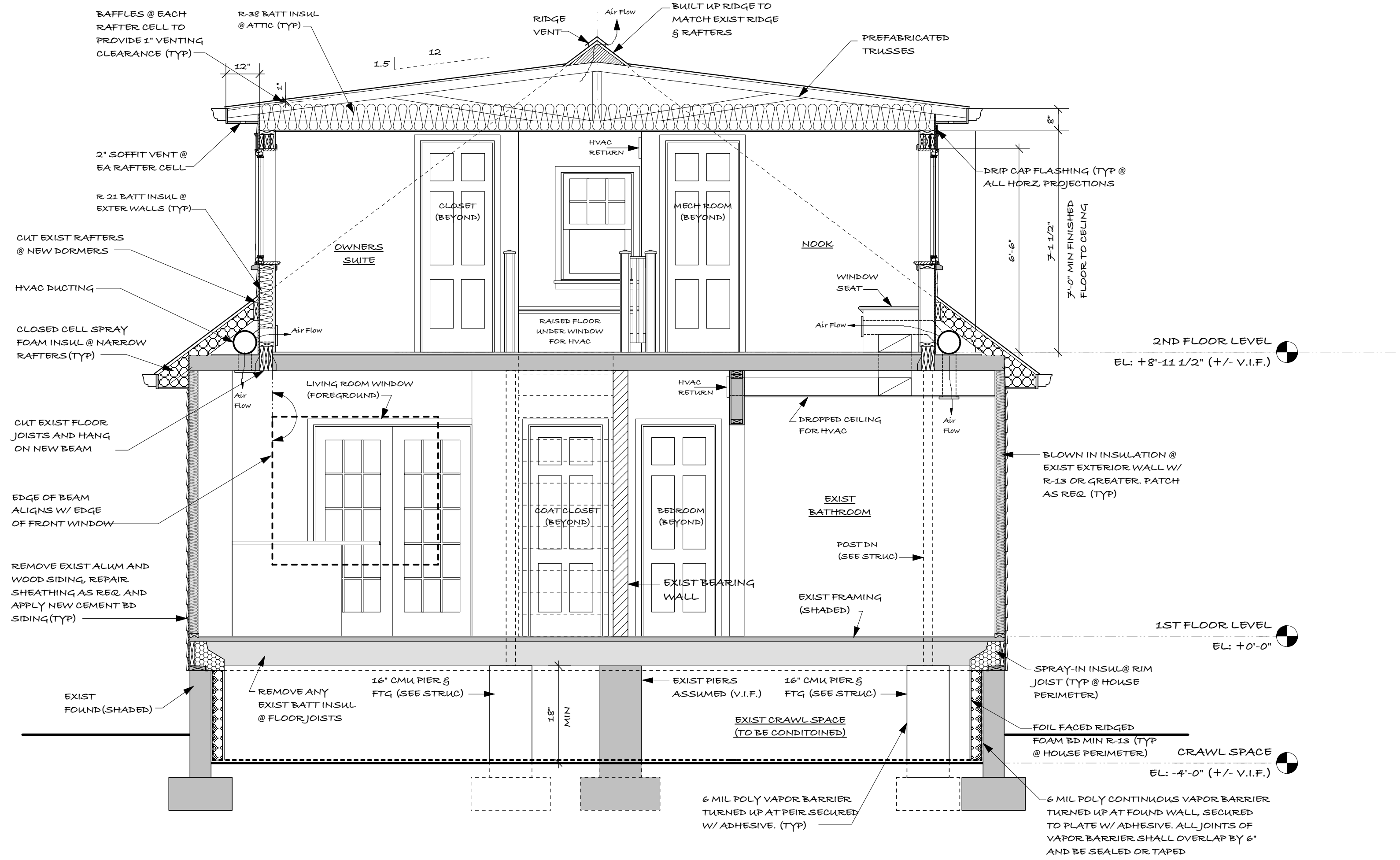
1 CROSS SECTION Scale: 3/8" = 1'-0"
